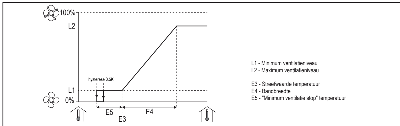
Afbeelding 2: Ventilatie niveau
