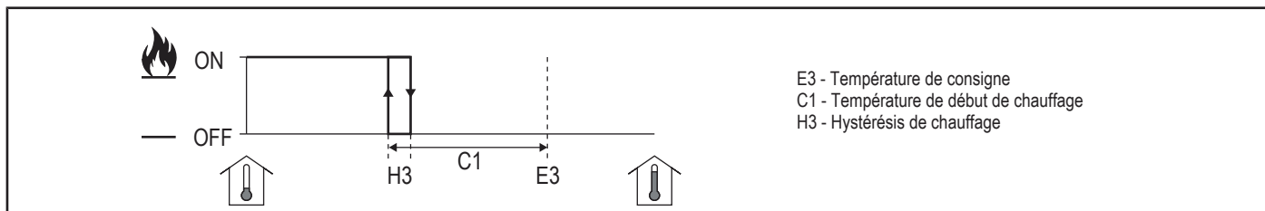
Fig. 6: Chauffage [ALLUMÉ / ÉTEINT]
