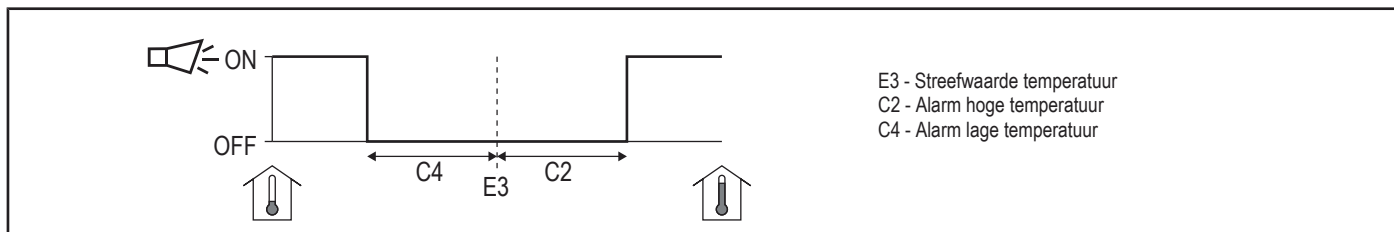
Afbeelding 8: Temperatuur alarmen
