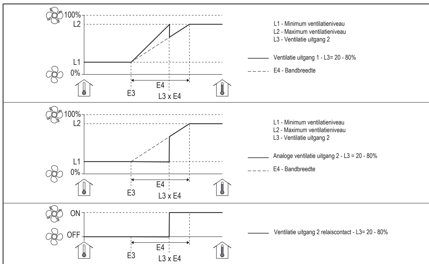
Afbeelding 3: Ventilatie uitgang 2 - [20 - 80%]
