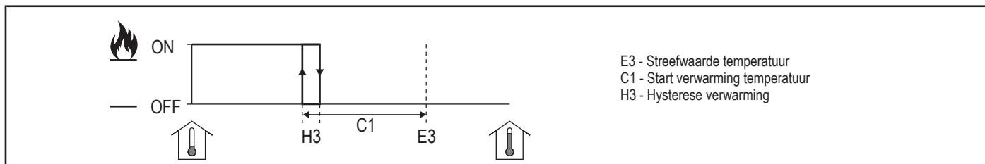
Afbeelding 6: Verwarming [AAN / UIT]
