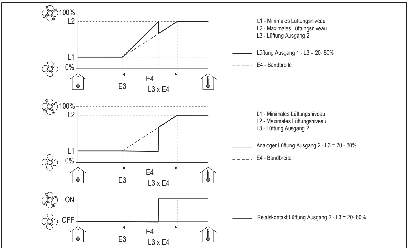
Abb. 3: Lüftung Ausgang 2 - [20 - 80%]
