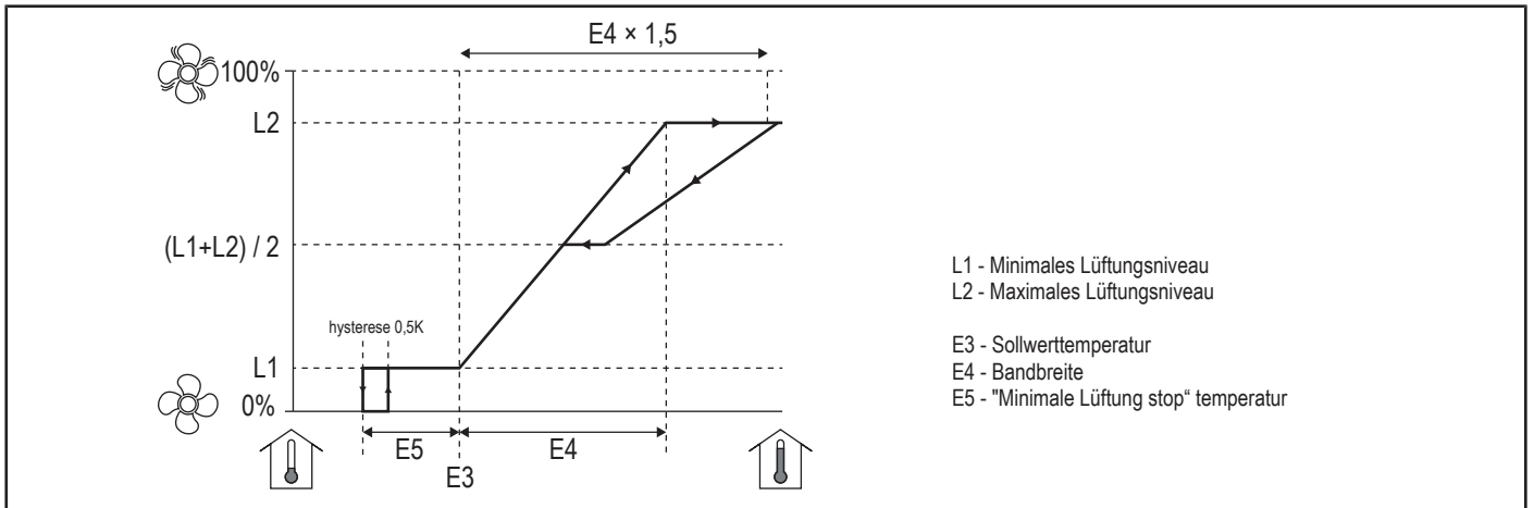
Abb. 4: Bandbreitenkompensation
