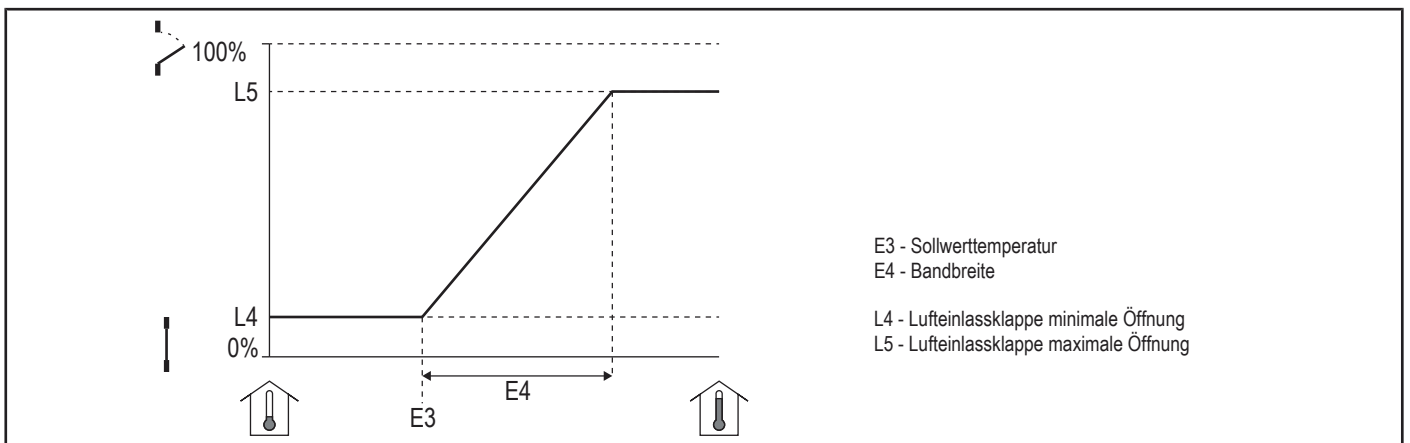
Abb. 5: Lufteinlassklappenöffnung [0 - 10 V]
