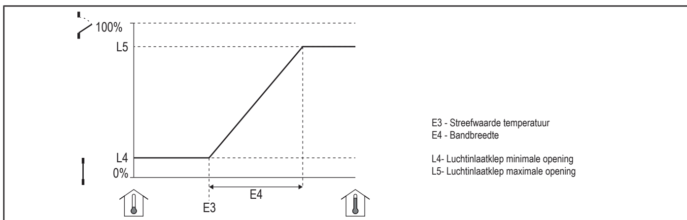
Afbeelding 5: Luchtinlaatklep opening [0-10 V]
