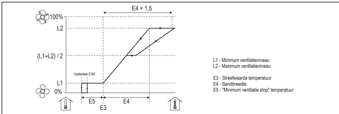
Afbeelding 4: Bandbreedtecompensatie
