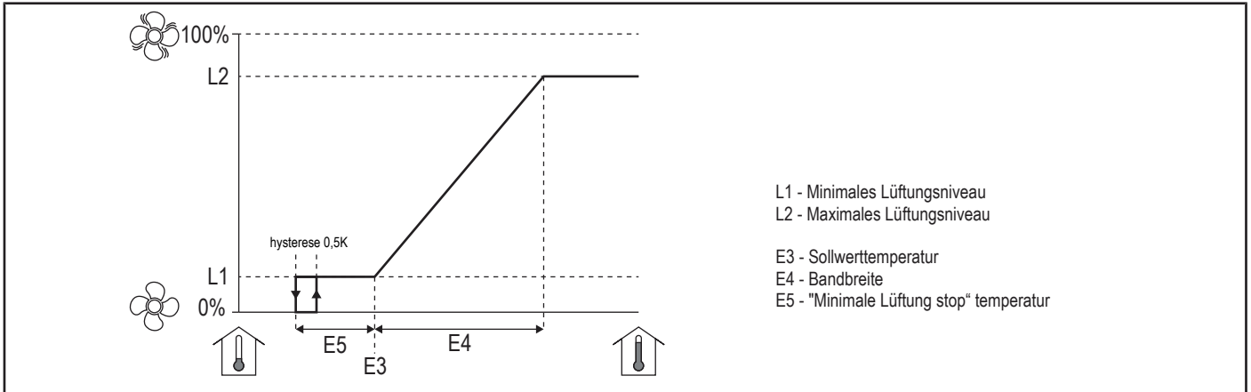
Abb. 2: Lüftungsniveau
