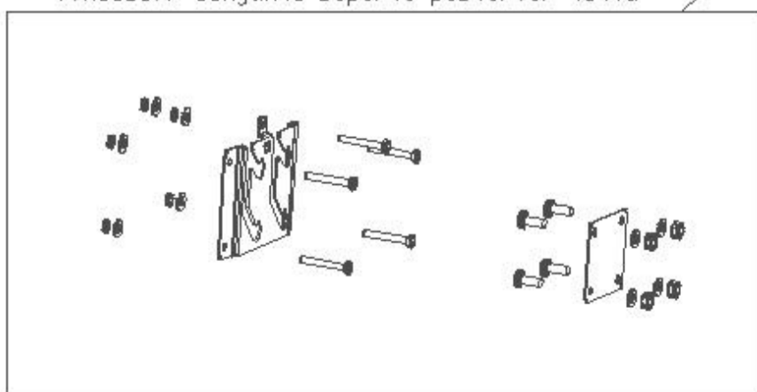
(TR5DB17) Conjunto soporte posterior tolva
