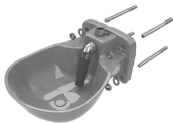
Seinäkiinnitys
